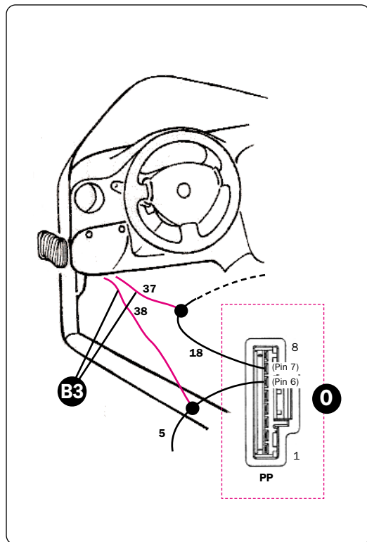
VISTA ANTERIORE DELLA CENTRALINA DI DERIVAZIONE - FRONT VIEW OF THE BRANCH UNIT VISTA ANTERIOR DE LA CENTRALITA DE DERIVACION - VISTA ANTERIOR UNIDADE CENTRAL DE DERIVAÇÃO ΜΕΤΩΠΙΑΚΗ ΟΨΗ ΤΟΥ ΚΕΝΤΡΙΚΟΥ ΠΡΟΒΛΕΥΣΗΣ - VUE AVANT DE LA CENTRALE DE DERIVATION ANSICHT VORDERSEITE STEUERINHEIT - A DERIVACIÓS KÖZPONT ELŐLNÉZETE PREDNÝ POHLAD NA DERIVAČNÚ JEDNOTKU - WIDOK PRZEDNI CENTRALKI ODGALEZIEN PŘEDNÍ POHLAD NA DERIVAČNÍ JEDNOTKU
