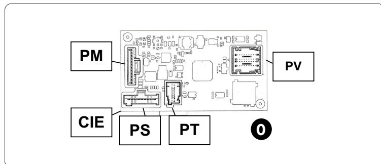
VISTA POSTERIORE DELLA CENTRALINA DI DERIVAZIONE - REAR VIEW OF THE BRANCH UNIT VISTA POSTERIOR DE LA CENTRALITA DE DERIVACION - VISTA POSTERIOR UNIDADE CENTRAL DE DERIVAÇÃO ΟΠΙΣΘΙΑ ΟΨΗ ΤΟΥ ΚΕΝΤΡΙΚΟΥ ΠΡΟΒΛΕΥΣΗΣ - VUE ARRIERE DE LA CENTRALE DE DERIVATION ANSICHT RÜCKSEITE STEUERINHEIT - A DERIVACIÓS KÖZPONT HÁTULNÉZETE ZADNÝ POHLAD NA DERIVAČNÚ JEDNOTKU - WIDOK TYLNY CENTRALKI ODGALEZIEN ZADNÍ POHLAD NA DERIVAČNÍ JEDNOTKU
