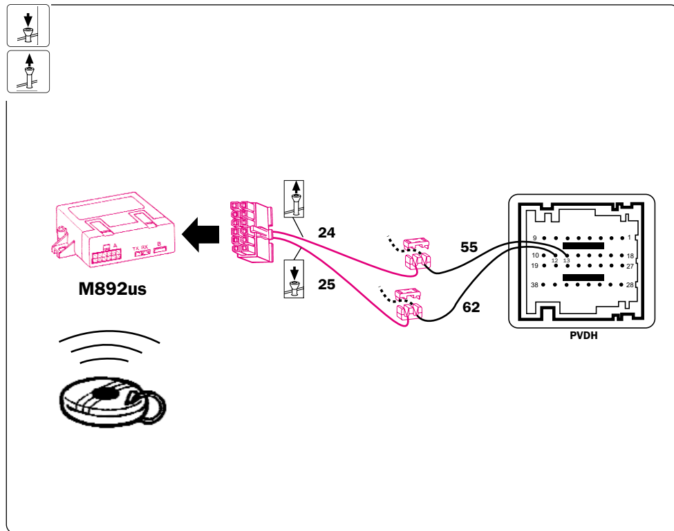
VISTA POSTERIORE DELLA CENTRALINA DI DERIVAZIONE - REAR VIEW OF THE BRANCH UNIT VISTA POSTERIOR DE LA CENTRALITA DE DERIVACION - VISTA POSTERIOR UNIDADE CENTRAL DE DERIVAÇÃO ΟΠΙΣΘΙΑ ΟΨΗ ΤΟΥ ΚΕΝΤΡΙΚΟΥ ΠΡΟΒΛΕΥΣΗΣ - VUE ARRIERE DE LA CENTRALE DE DERIVATION ANSICHT RÜCKSEITE STEUERINHEIT - A DERIVACIÓS KÖZPONT HÁTULNÉZETE ZADNÝ POHLAD NA DERIVAČNÚ JEDNOTKU - WIDOK TYLNY CENTRALKI ODGALEZIEN ZADNÍ POHLAD NA DERIVAČNÍ JEDNOTKU
