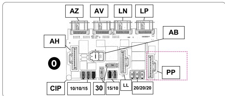
VISTA ANTERIORE DELLA CENTRALINA DI DERIVAZIONE - FRONT VIEW OF THE BRANCH UNIT VISTA ANTERIOR DE LA CENTRALITA DE DERIVACION - VISTA ANTERIOR UNIDADE CENTRAL DE DERIVAÇÃO ΜΕΤΩΠΙΑΚΗ ΟΨΗ ΤΟΥ ΚΕΝΤΡΙΚΟΥ ΠΡΟΒΛΕΥΣΗΣ - VUE AVANT DE LA CENTRALE DE DERIVATION ANSICHT VORDERSEITE STEUERINHEIT - A DERIVACIÓS KÖZPONT ELŐLNÉZETE PREDNÝ POHLAD NA DERIVAČNÚ JEDNOTKU - WIDOK PRZEDNI CENTRALKI ODGALEZIEN PŘEDNÍ POHLAD NA DERIVAČNÍ JEDNOTKU
